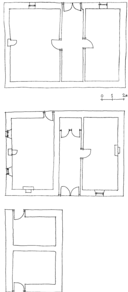
Сл.12. Основи на куќа од затворен тип во три нивоа, с.Белица, 19 ти век
