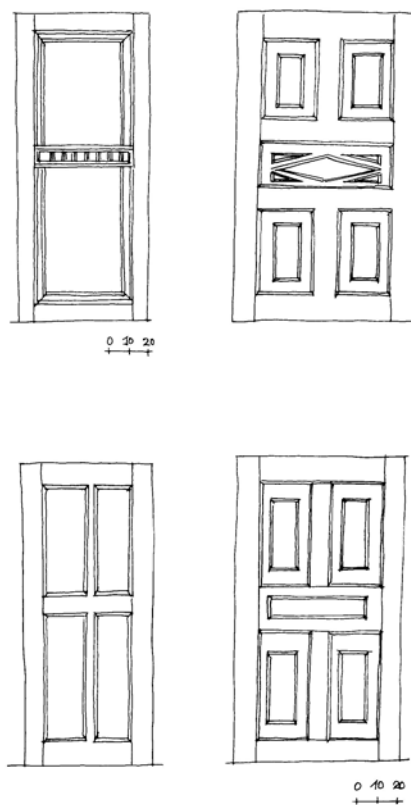
Сл.24. Изглед на внатрешни врати, с.Србјани, с.Кленоец, с.Иваништа
