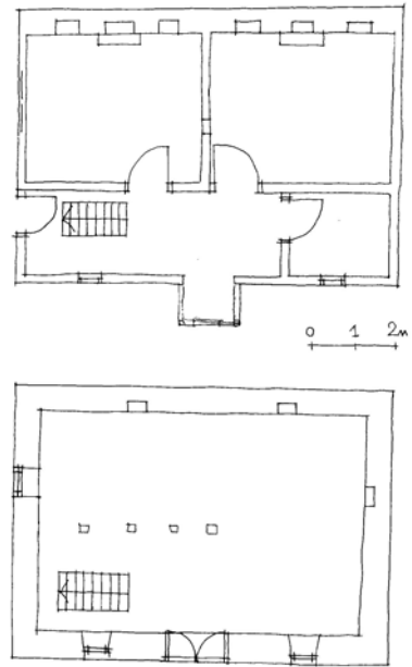
Сл.10. Основи на затворен тип на куќа со приземје и кат, с.Миокази, 19 ти век
