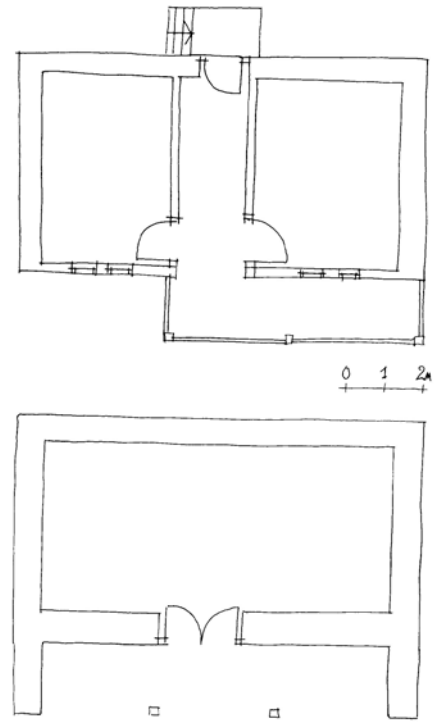
Сл.6. Основи на куќа во две нивоа со отворен чардак, странично поставен, с.Јудово, 19 ти век
